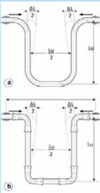
Fig. 12 Compressori di dilatazione ad "U" soto traccia
