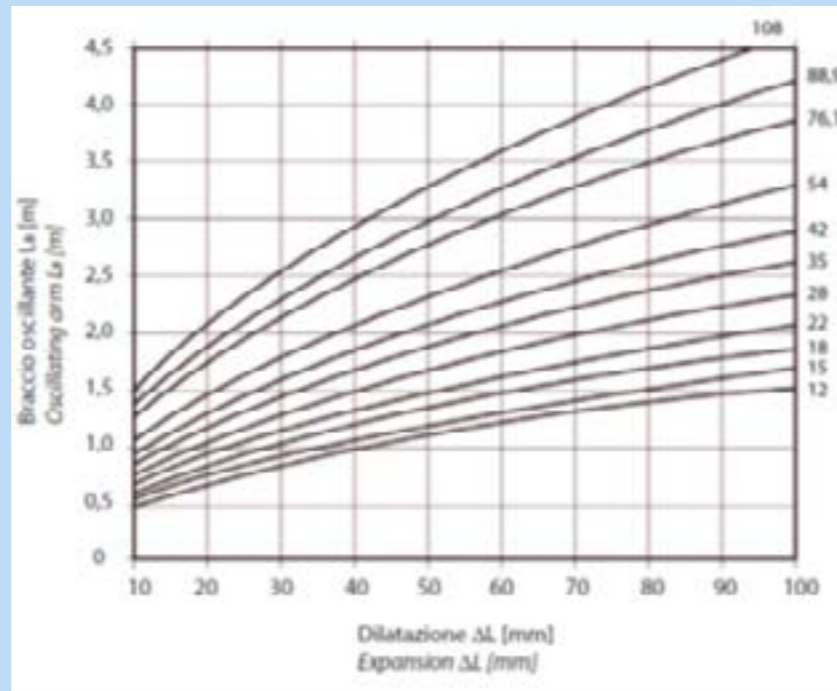
Fig. 16 lunghezza Le del compressore a Z in acciaio inossidabile
