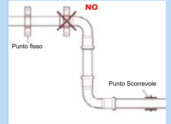
Fig. 19 Fissaggio delle tubazioni: punto fisso in corrispondenza del raccordo: errato.
